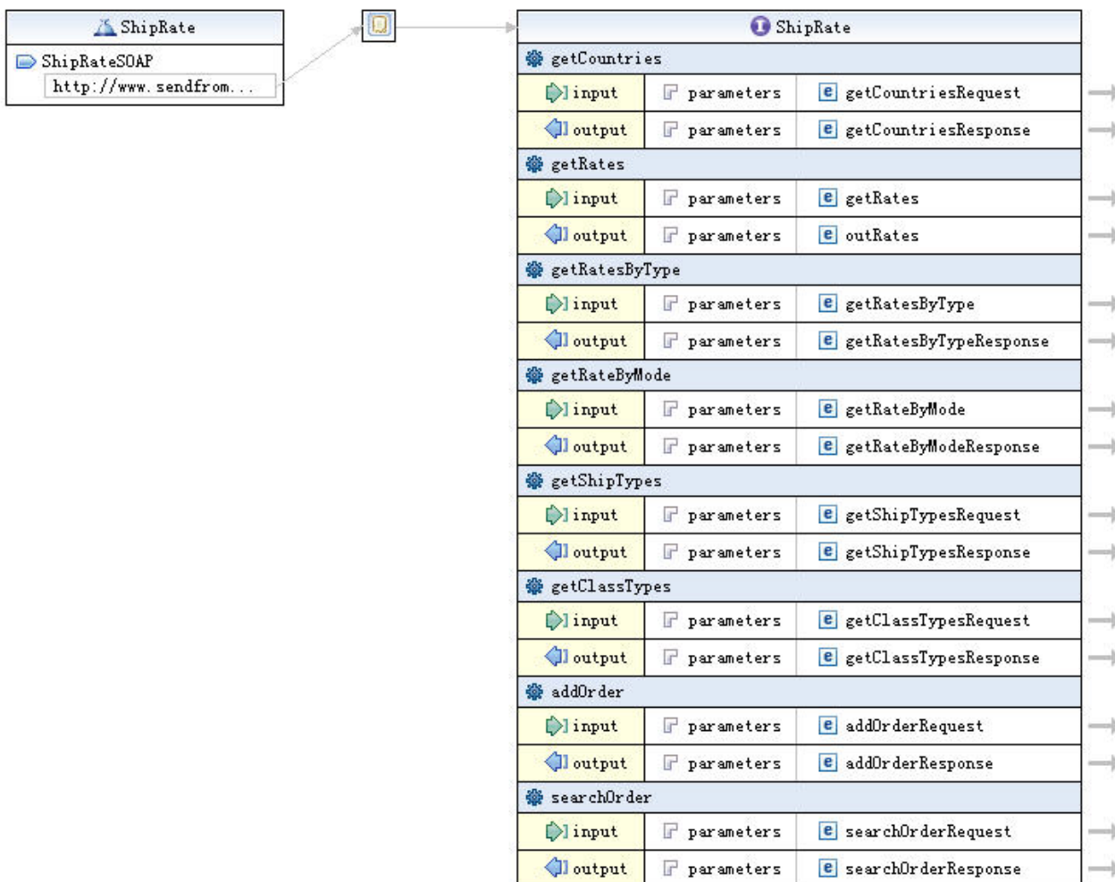
(结构图)
